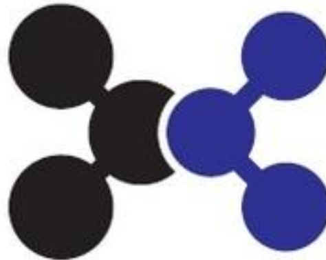
ИНКЛЮЗИВНАЯ МОЛЕКУЛА
